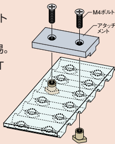
専用ナット
