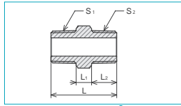
SRNニップル
