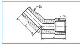
SHL45度めすおすエルボ
