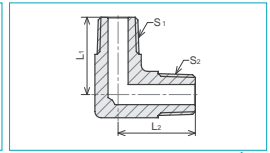
SMLおすエルボ
