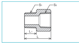
SXSめすおすソケット
