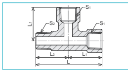
SRTめすおすティー
