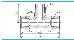
SXTめすおすティー
