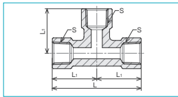
SFTめすティー
