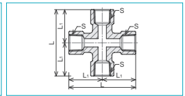
SFCめすクロス
