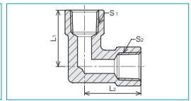
SFLめすエルボ
