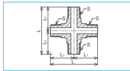
SMCおすクロス
