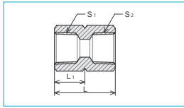
SFSめすソケット
