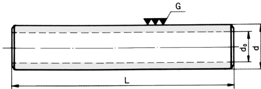
SFP型寸法図
