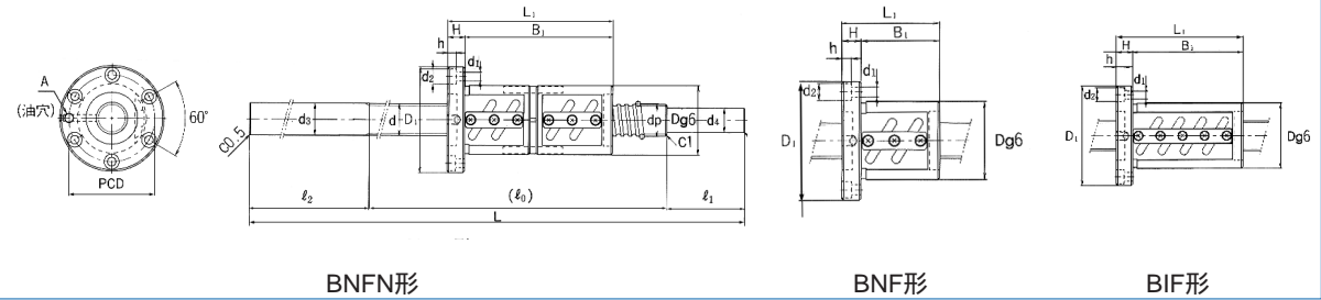
寸法図
