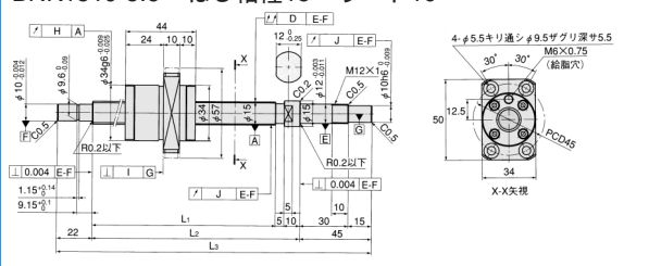
BNK1510-5.6 ねじ軸径15 リード10
