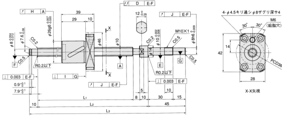
BNK1205-2.5 ねじ軸径12,リード5
