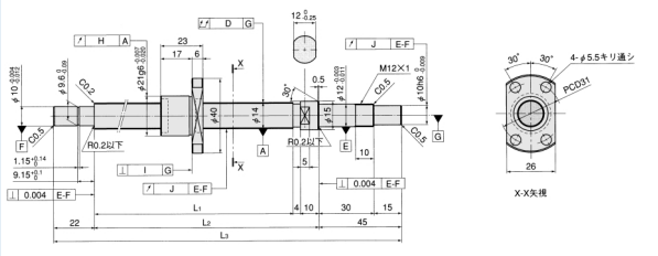
BNK1408-2.5 ねじ軸径14,リード8
