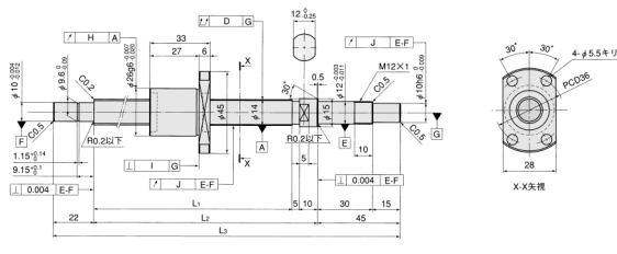
BNK1404-3 ねじ軸径14,リード4
