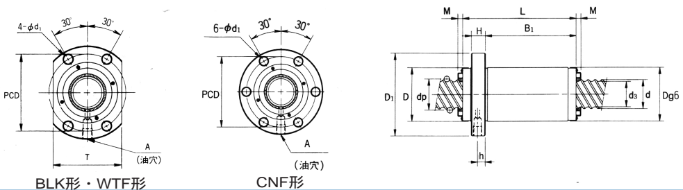
寸法図
