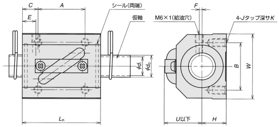
RNSTL形寸法図
