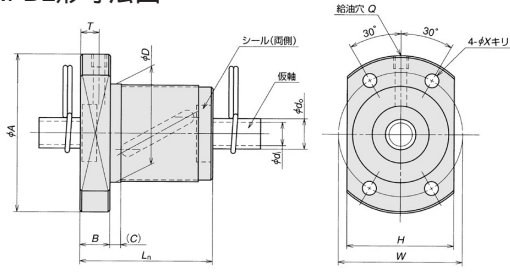
RNFBL形寸法図
