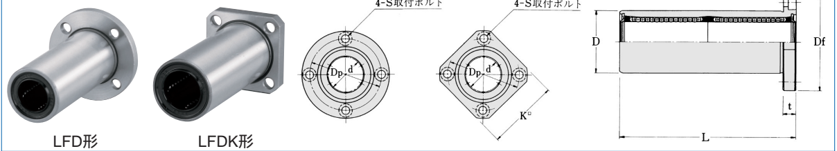
寸法図
