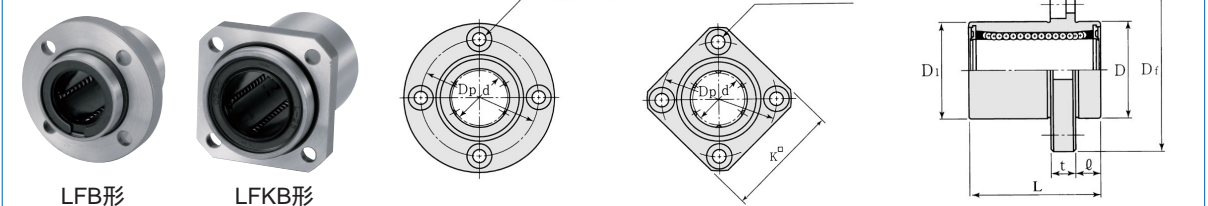
寸法図
