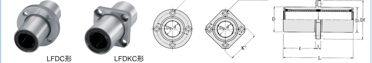
寸法図
