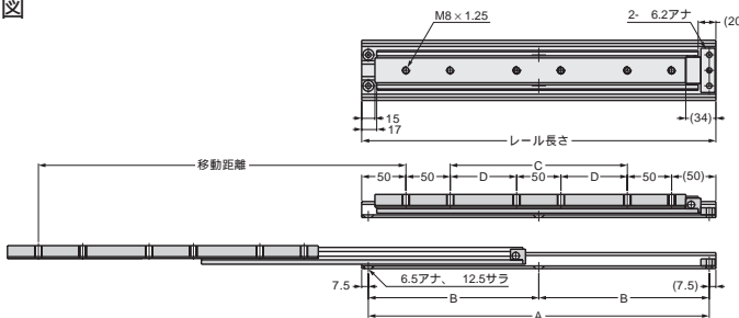
CBL-RA7R型スライドレール(耐荷重340～130kg)完全スライド 自重：8kg/m
