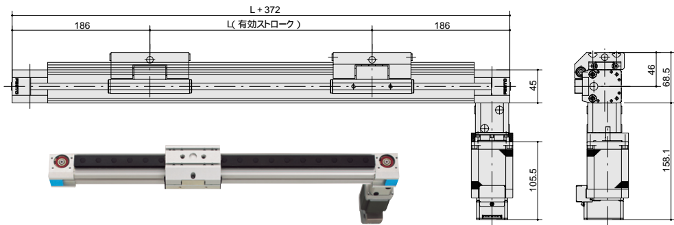
BGA25型寸法図
