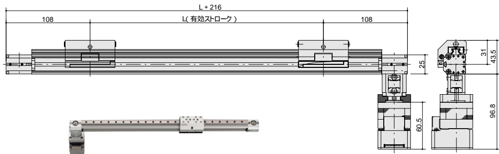
BGA12型寸法図
