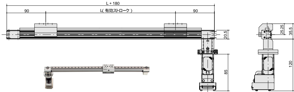
BGA08型寸法図
