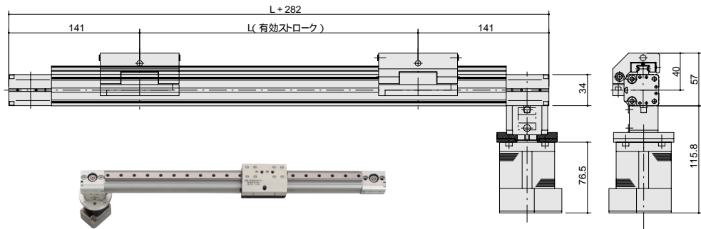
BGA18型寸法図
