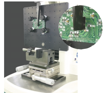
はんだ付強度試験 (治具はオプションです)
