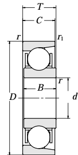
EN形寸法図
