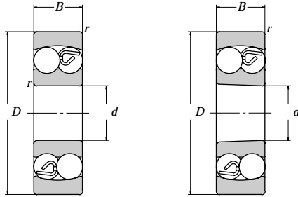
円筒穴
