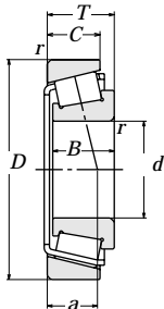
HR30300D形価格寸法表
