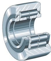
NUTR形 (INA理想外径形状)
