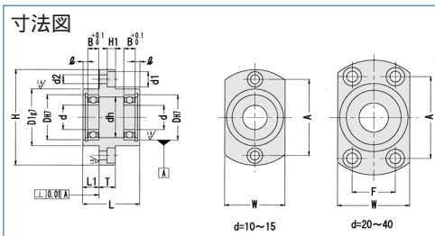
DEIS型 (SUS)
