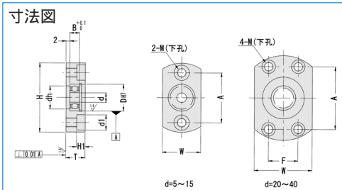
BERS型 (SUS)
