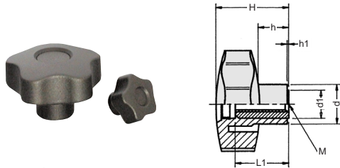
STK-N形
