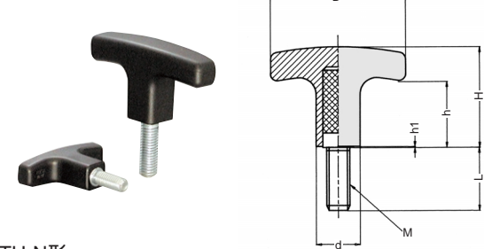
TH-N形 ノブ: 黒色ナイロン樹脂 (ガラス繊維強化) ネジ: SUM22L 三価クロメート TH-N形ティーハンドル
