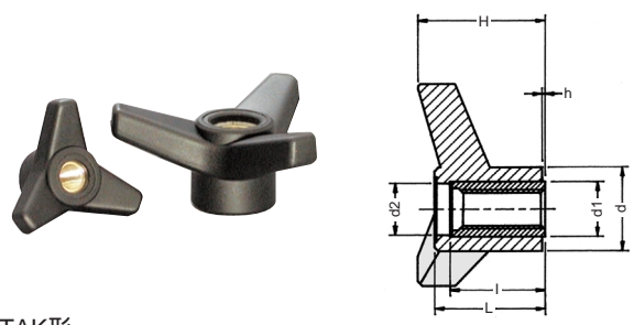
TAK形 ノブ: 黒色ナイロン樹脂 (ガラス繊維強化) インサート: 黄銅 TAK形スリーアームノブ
