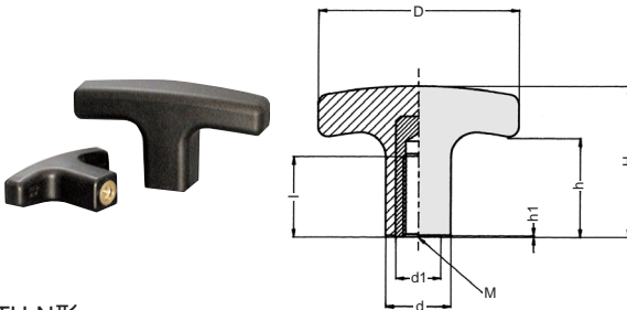
TH-N形 ノブ: 黒色ナイロン樹脂 (ガラス繊維強化) インサート: 黄銅 TH-N形ティーハンドル
