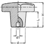
Cタイプ Rタイプ CK形クロスノブ
