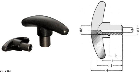
TH形 ノブ: 黒色フェノール樹脂、インサート: SUM22L 黒色四三酸化鉄皮膜 TH形ティーハンドル
