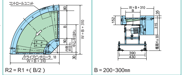
寸法図(SMBM形)
