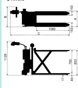
寸法図
