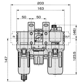
W2000外形寸法
