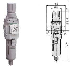
F2000外形寸法
