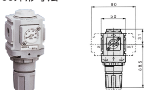
R2000外形寸法
