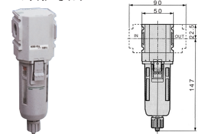
R2000外形寸法
