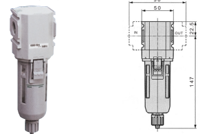
M2000外形寸法
