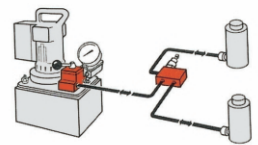
ライン設置タイプ
