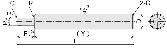
SPD型、SPSD型寸法図
