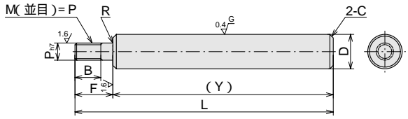
SPO型、SPSO型寸法図
