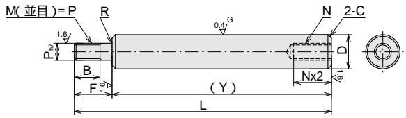
SPOM型、SPSOM型寸法図
