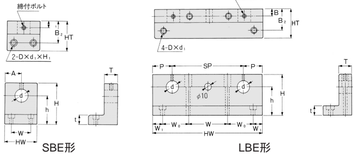
寸法図
