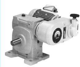
TW形(0.2~3.7kW)
