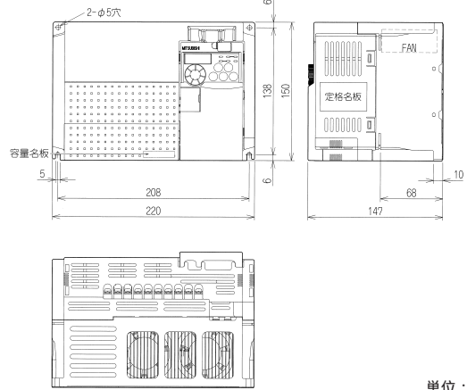
単位 : mm
