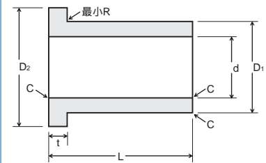
寸法図(フランジ付)
