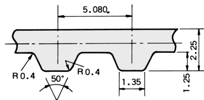
XL形標準歯形形状
