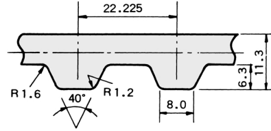
XH形標準歯形形状
