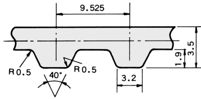
L形標準歯形形状
