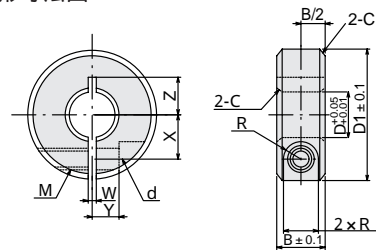
RSB-MS形寸法図
