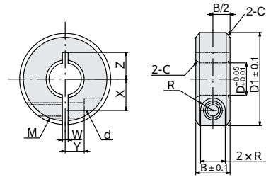
RSB形寸法図
