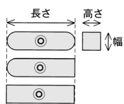
抜きタップ両丸キー、片丸キー、両角キー寸法図
