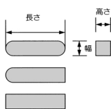
両丸キー、片丸キー、両角キー寸法図
