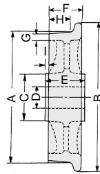
寸法図
