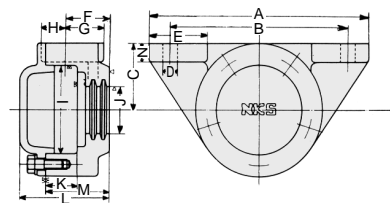
寸法図
