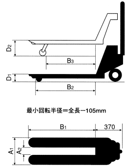
寸法図
