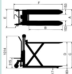
LV50寸法図
