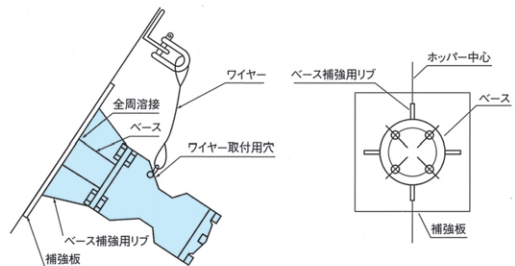
取付方法
