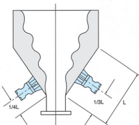
取付例
