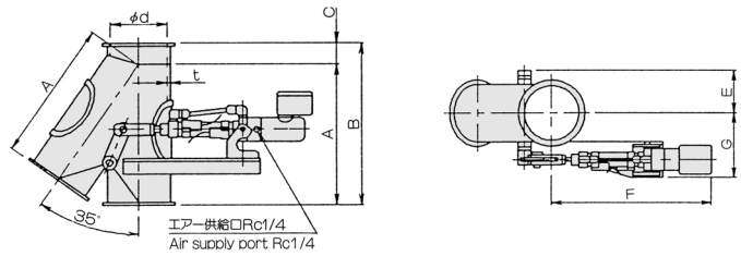
寸法図
