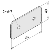
② 直線プレート
