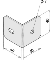
③ 90°プレート
