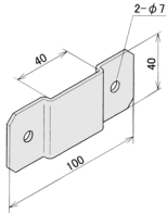
① 連結プレート
